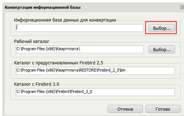
Рисунок 12 – Выбор информационной базы для конвертации
